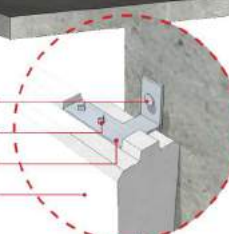
Gb. 1 Pemasangan LeichtPanel diluar Struktur
